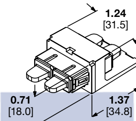
Mini-Com® SC Duplex Adapter Module
